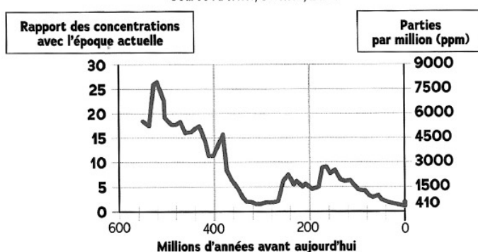
fig. 3 Évolution du CO2 dans le temps
