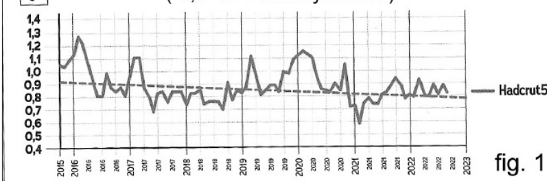
Evolution de la température terrestre de 2015 à 2023 (-0,1° C° : Hadley Center)
