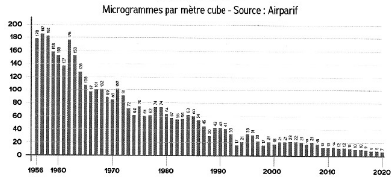
fig. 2 Évolution globale des particules dans l'agglomération parisienne 1956-2020
